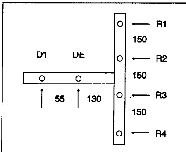
Bild/Figure 6: Reflector-Arrangement for BV-Series
